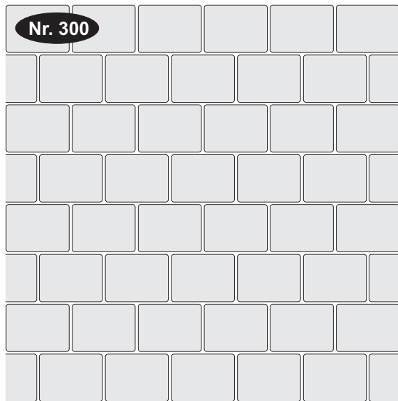
Halbverband mit Stein 240/180
