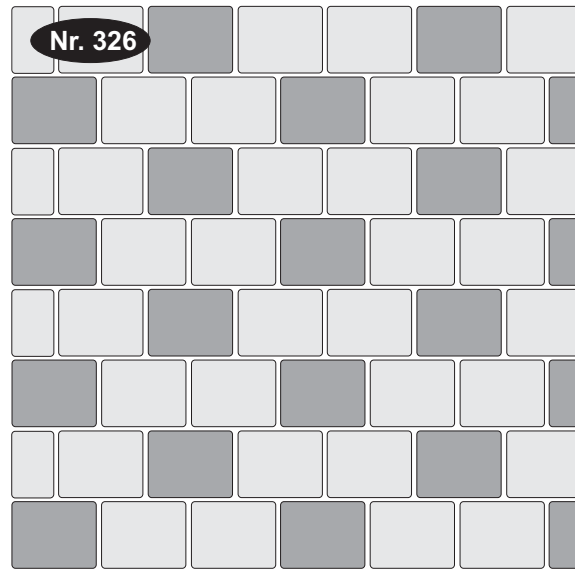
Halbverband mit Stein 240/180 in zwei Farben
