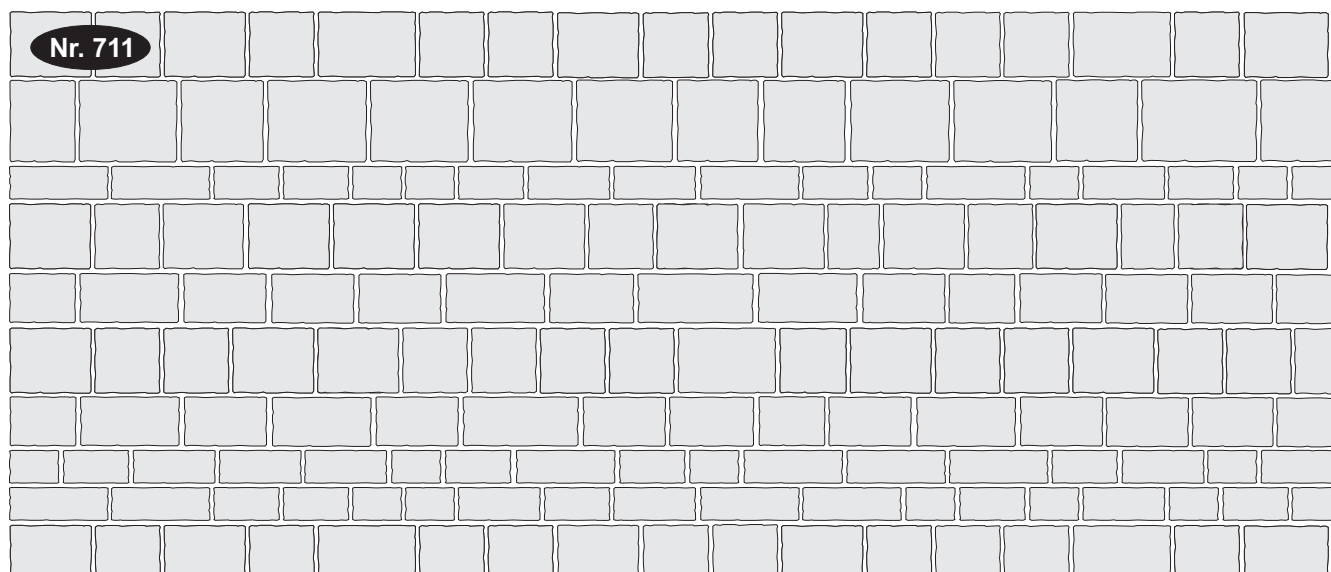
Reihenverband mit den 16 Steinen der Sortimente 80, 120, 160 und 200
