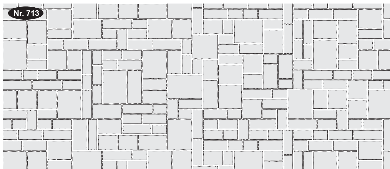
Römischer Verband mit den 16 Steinen der Sortimente 80, 120, 160 und 200 (mit höherem Anteil des Sortiments 80)
