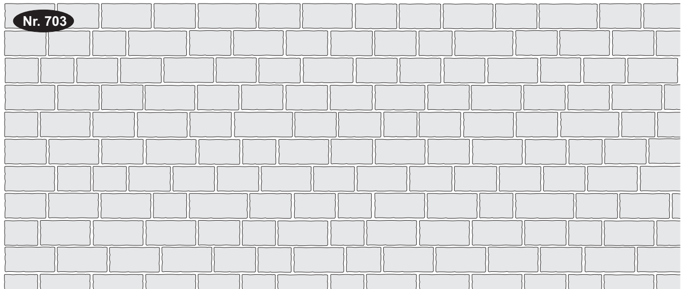
Läuferverband mit den 4 Steinen des Sortiments 120
